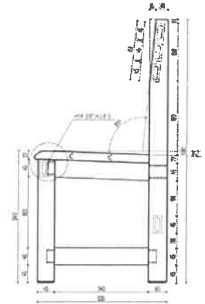
VISTA LATERAL Escala 1/4
