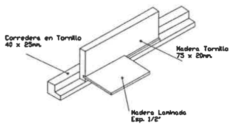
DETALLE CAJONERIA
