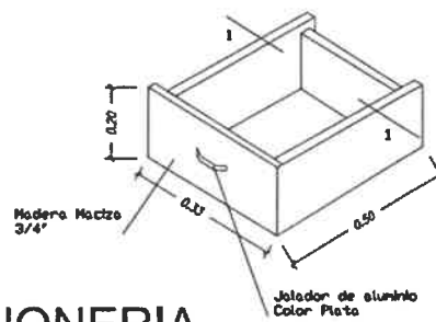
DETALLE CAJONERIA
