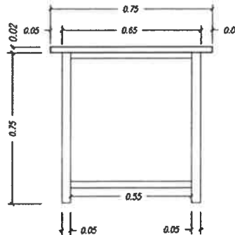
ELEVACIÓN LATERAL
