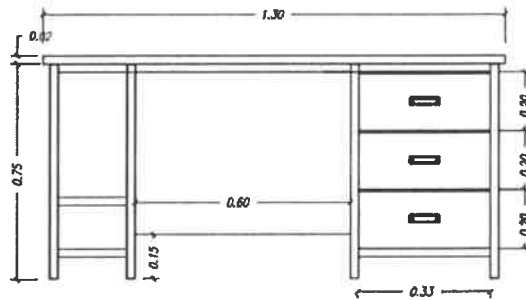
ELEVACIÓN PRINCIPAL
