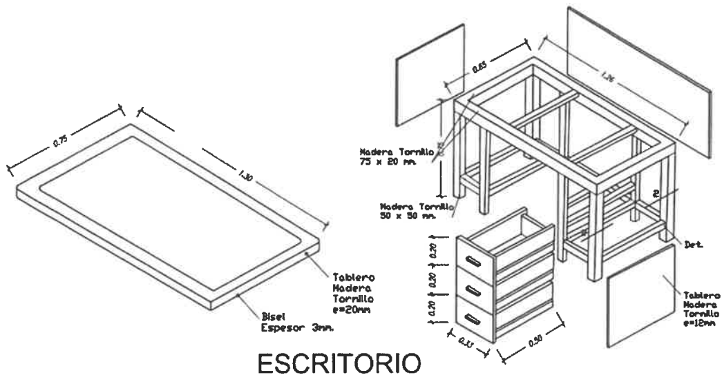
ISOMETRICO DE ESCRITORIO
