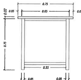
ELEVACIÓN LATERAL
