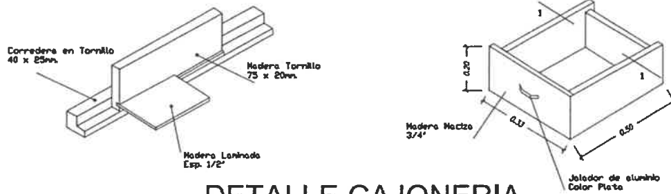
DETALLE CAJONERIA
