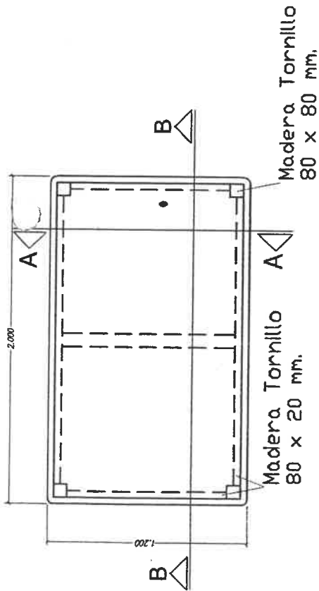
PLANTA
