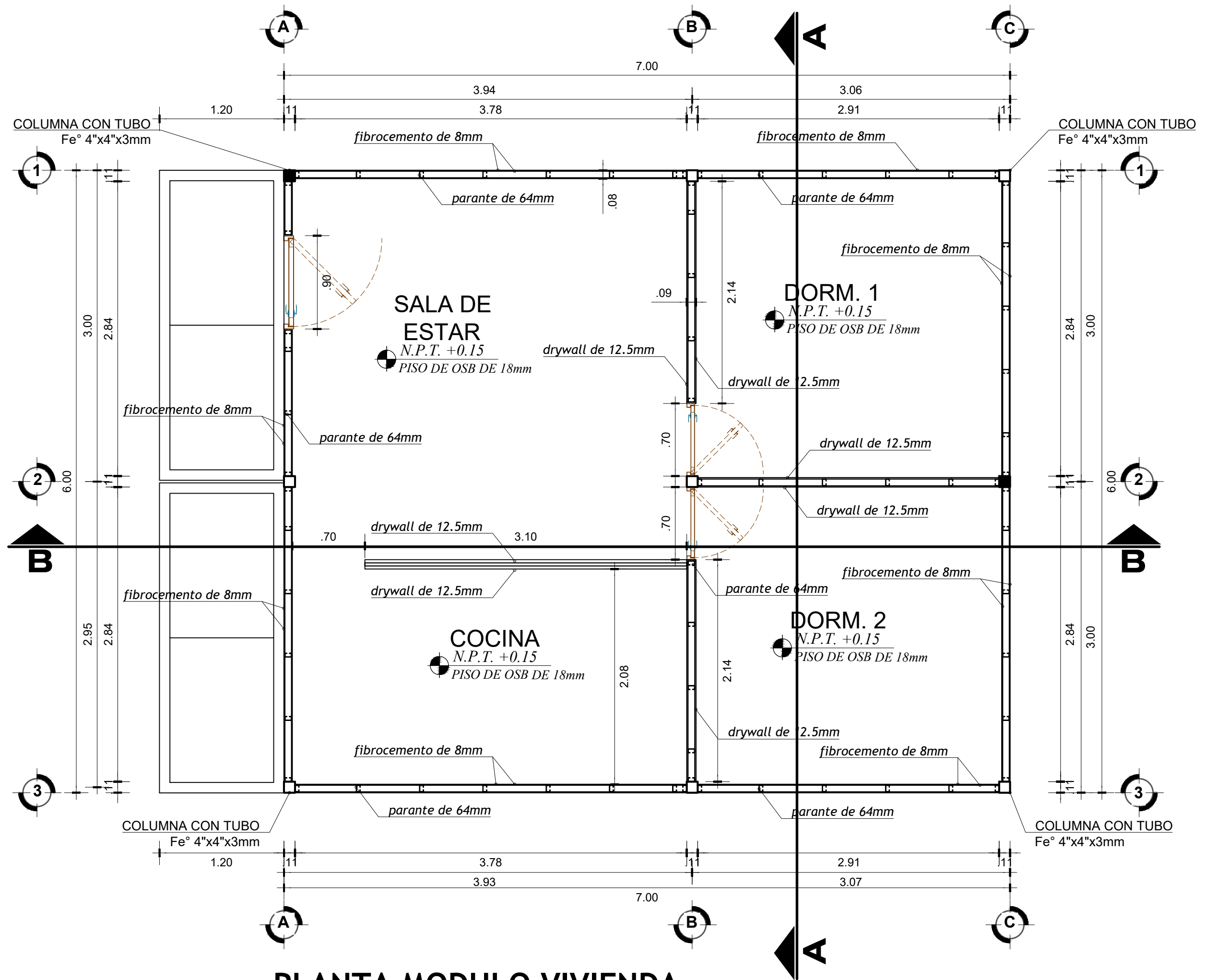
PLANTA MODULO VIVIENDA ESC: 1/50
