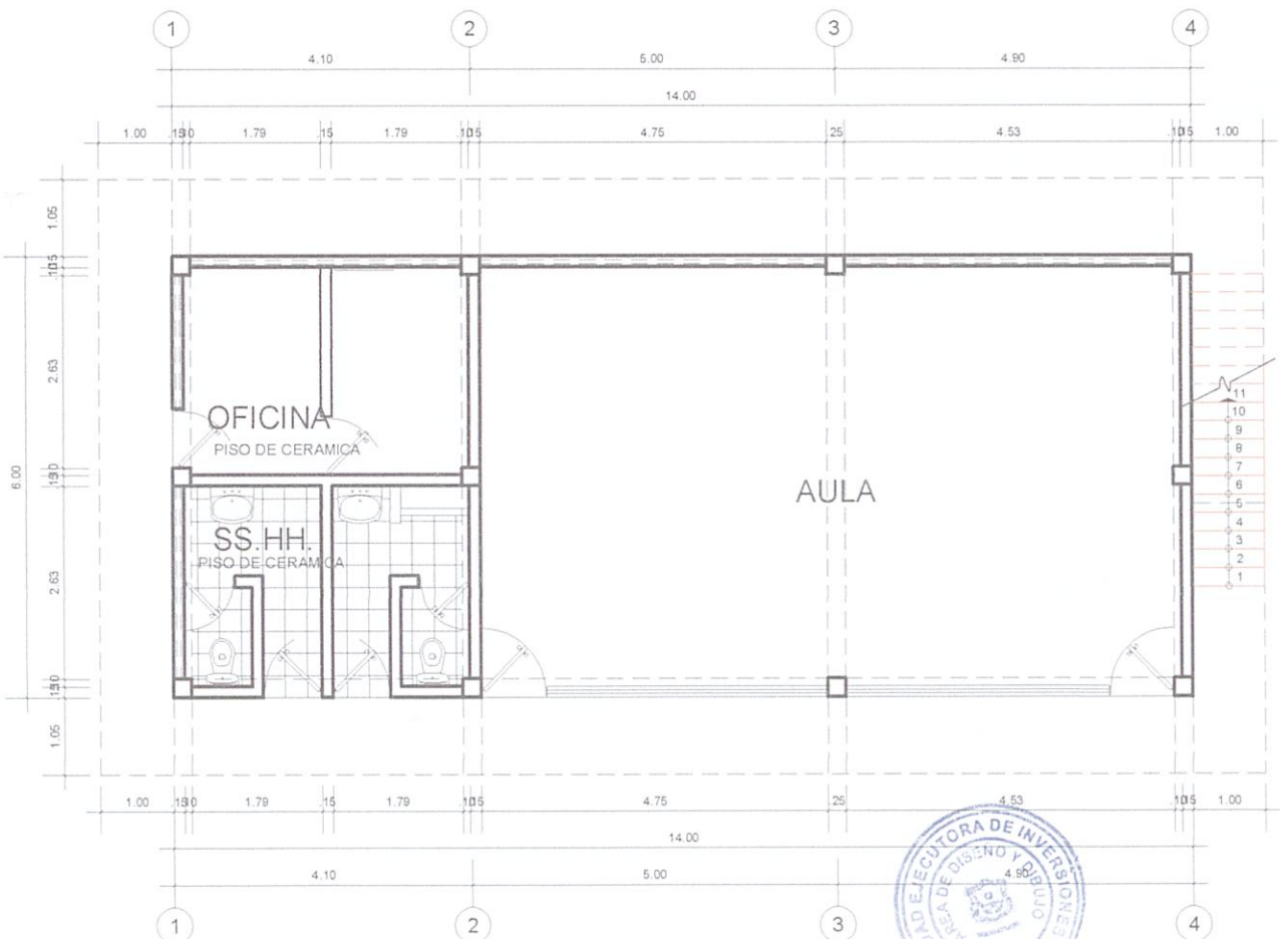
PLANTA PRIMER PISO ESC. 1/125
