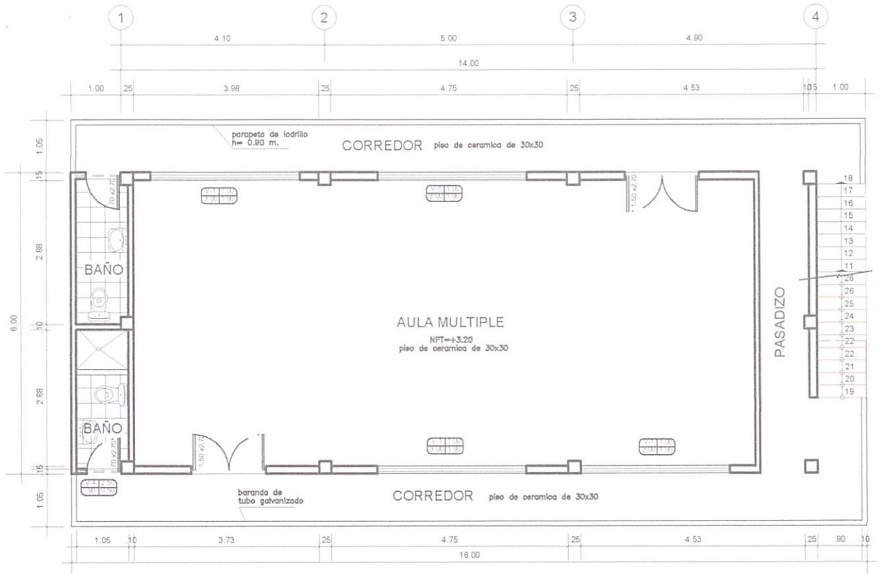
PLANTA SEGUNDO PISO ESC. 1/75
